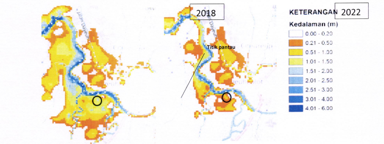
Sumber: Pemodelan Pusair dan BBWS Gambar 5.29 Perbandingan Kedalaman Untuk Kondisi Tahun 2018 ( Basecase ) dan Tahun 2022
