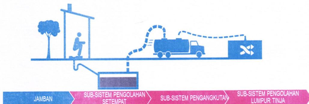
Gambar 5.15 Alur Kegiatan Air Limbah SPALD Setempat
