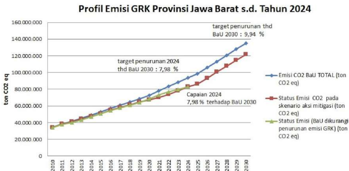
Gambar 4.8 Profil Emisi Gas Rumah Kaca Provinsi Jawa Barat
