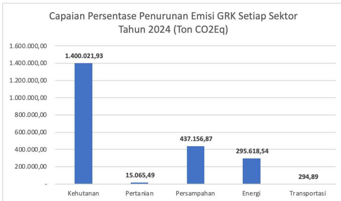
Gambar 4.9 Kontribusi Capaian Penurunan Emisi Gas Rumah Kaca setiap Sektor Tahun 2024
